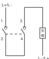
单极接地系统
