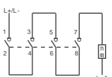
单极接地系统
