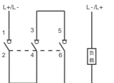
单极接地系统
